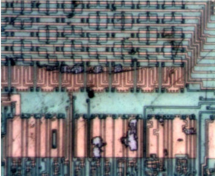
Koaxiale Kaltlichtbeleuchtung (Schwanenhals)
